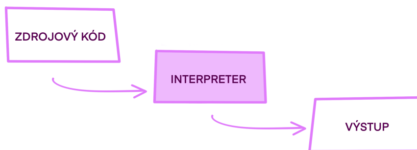
Obr. 1.8: Interpreter
