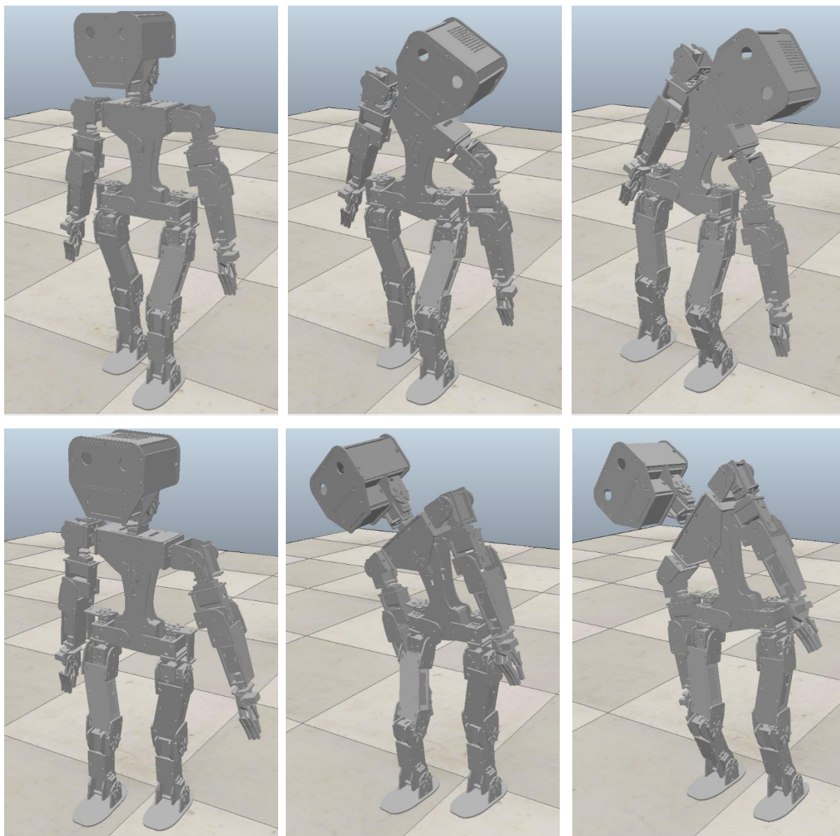
Obrázok 9 Šesť polôh tvoriacich chôdzu
